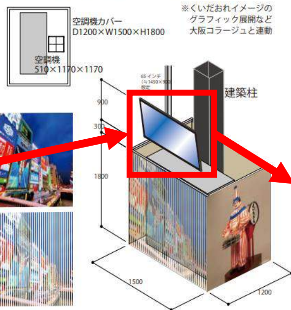
空調機の柱間き造作壁面イメージ例
